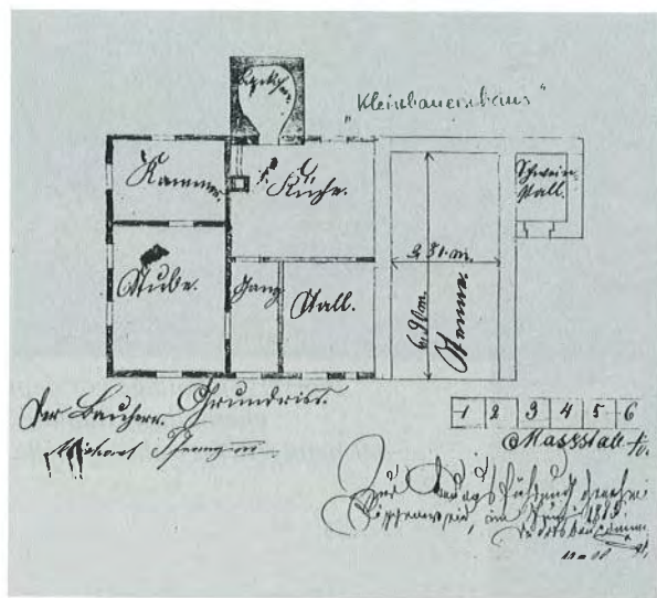
Haus des Michael Pfrang III., 1895. Der Wohnteil liegt links.
